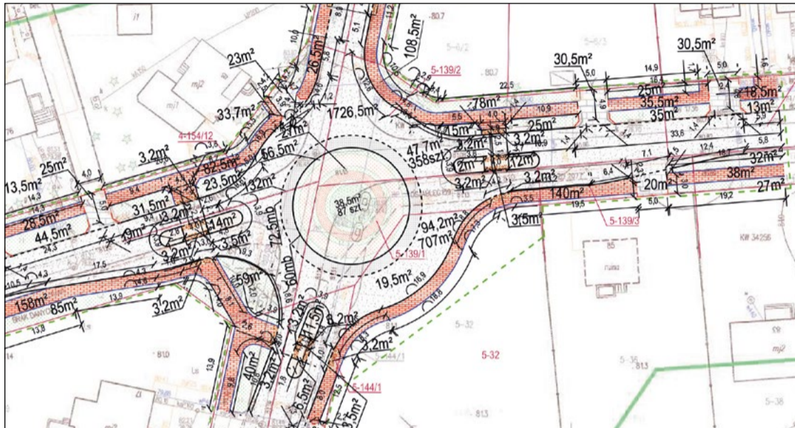
Projekt budowlany planowanego ronda
